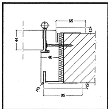
Particolare Telaio R3
